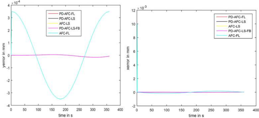
(d) y track errors of all controllers except PD
