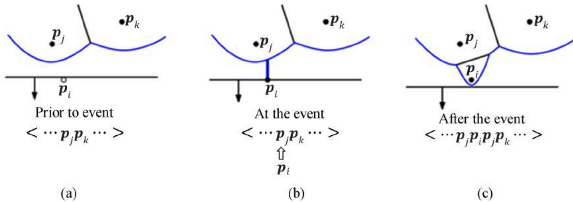
Fig. 6. Site event.
