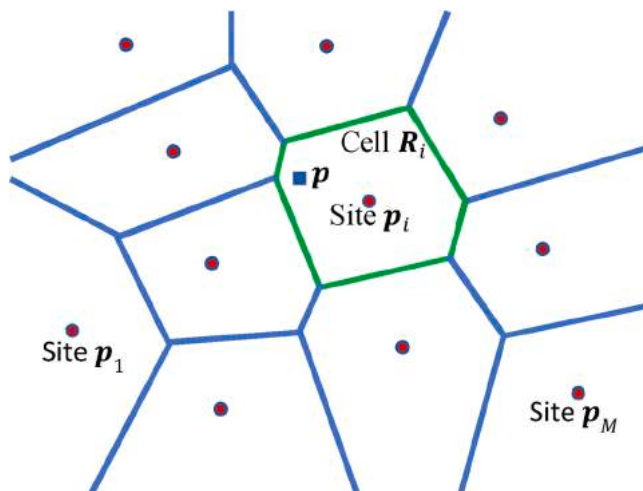
Fig. 4. Voronoi diagram.
