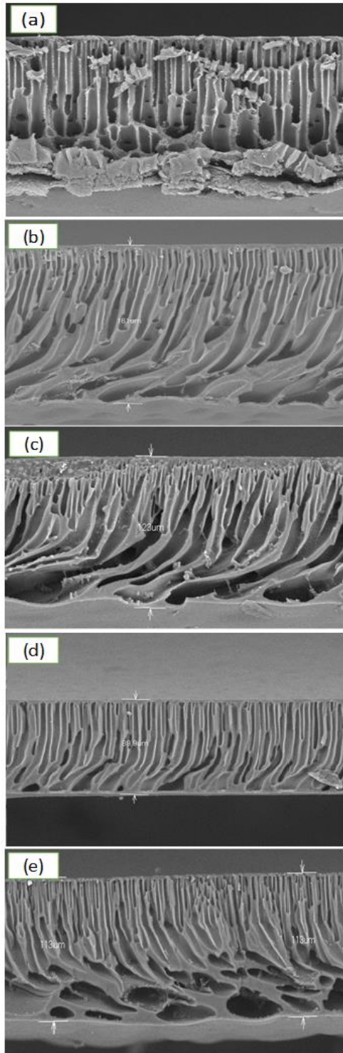
Figure 2 SEM images (a) P84 polymeric membrane (b) CM-600°C, (c) CM-700°C, (d) CM-800°C (e) CM-900 °C
