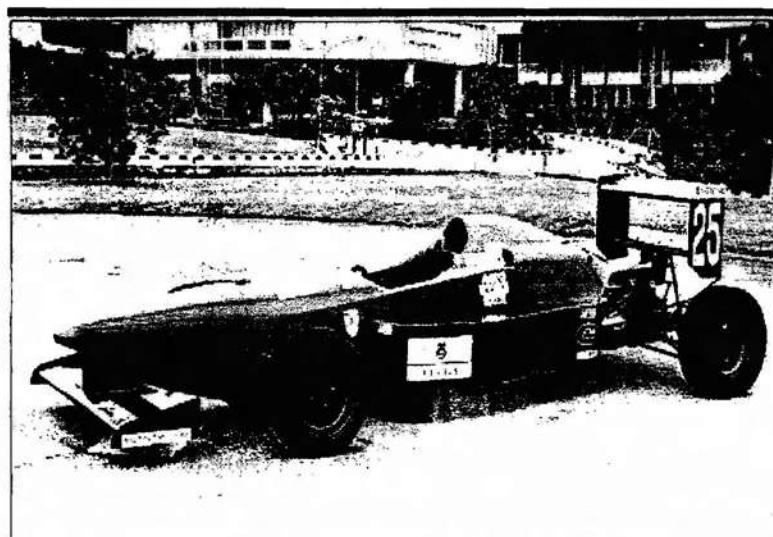
Rajah 17 Prototaip Formula-M yang Telah Siap Sepenuhnya
