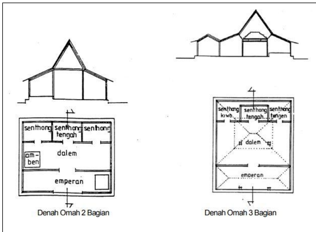
Gambar foto 1.4 Contoh ruangan dalam rumah tradisional Jawa (Alfari, 2017)
