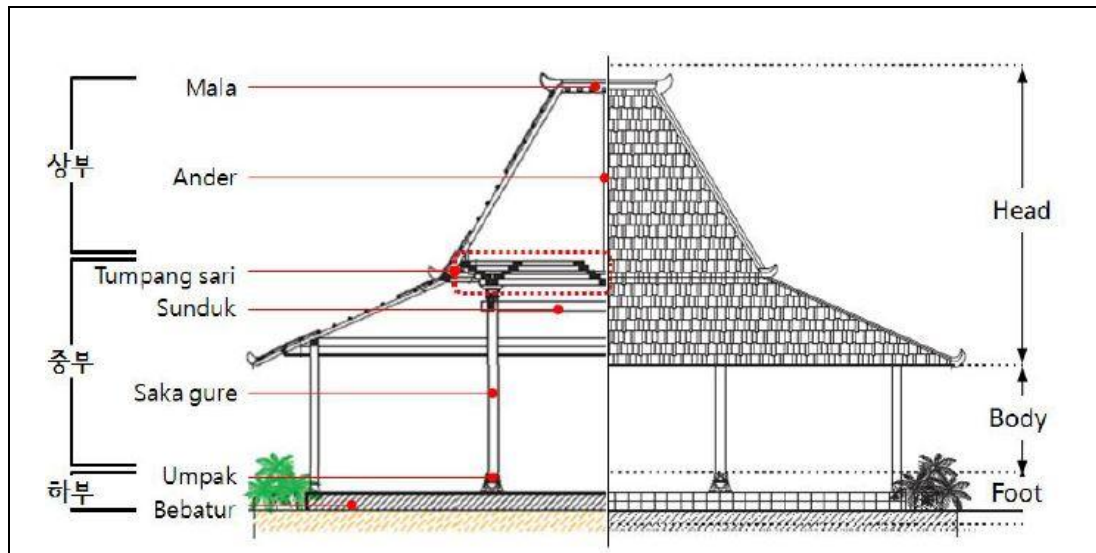
Gambar rajah 1.5 Pembahagian ruang secara horizontal bagi rumah tradisional Jawa (Do-Yeon, Hye-Kyung, & Seo-Ryeong, 2013)
