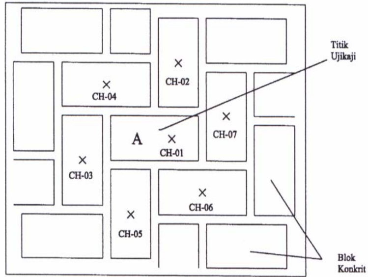
Rajah 4 : Kedudukan Cerapan Tranduser Pada Titik A
