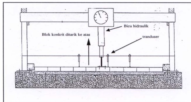
Rajah 3 : Keratan Rentas Kerangka Ujian Tarik Keluar
