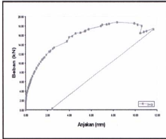
Rajah 6 : Graf Beban (kN) Melawan Anjakan (mm) (Pull Out ~ CH-02)
