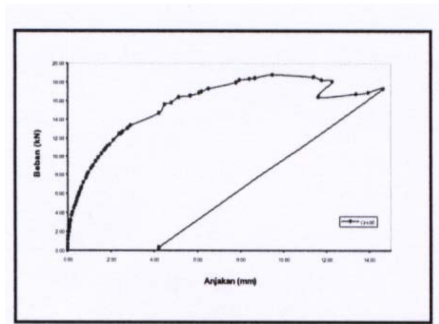
Rajah 10 : Graf Beban (kN) Melawan Anjakan (mm) ( Pull Out ~ CH-06 )
