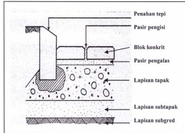
Rajah 2 : Lapisan Turapan Blok Konkrit
