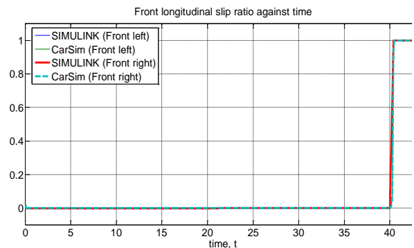
(d) Front longitudinal slip against time
