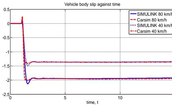
(d) Vehicle body slip against time
