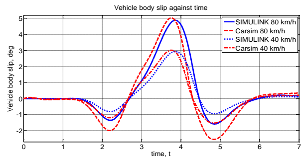
(d) Vehicle body slip against time
