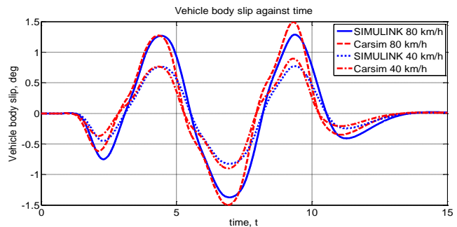
(d) Vehicle body slip against time
