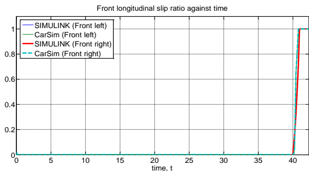
(d) Front longitudinal slip against time
