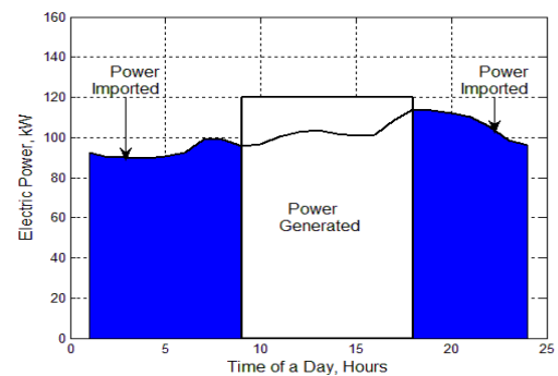
a) No TES
